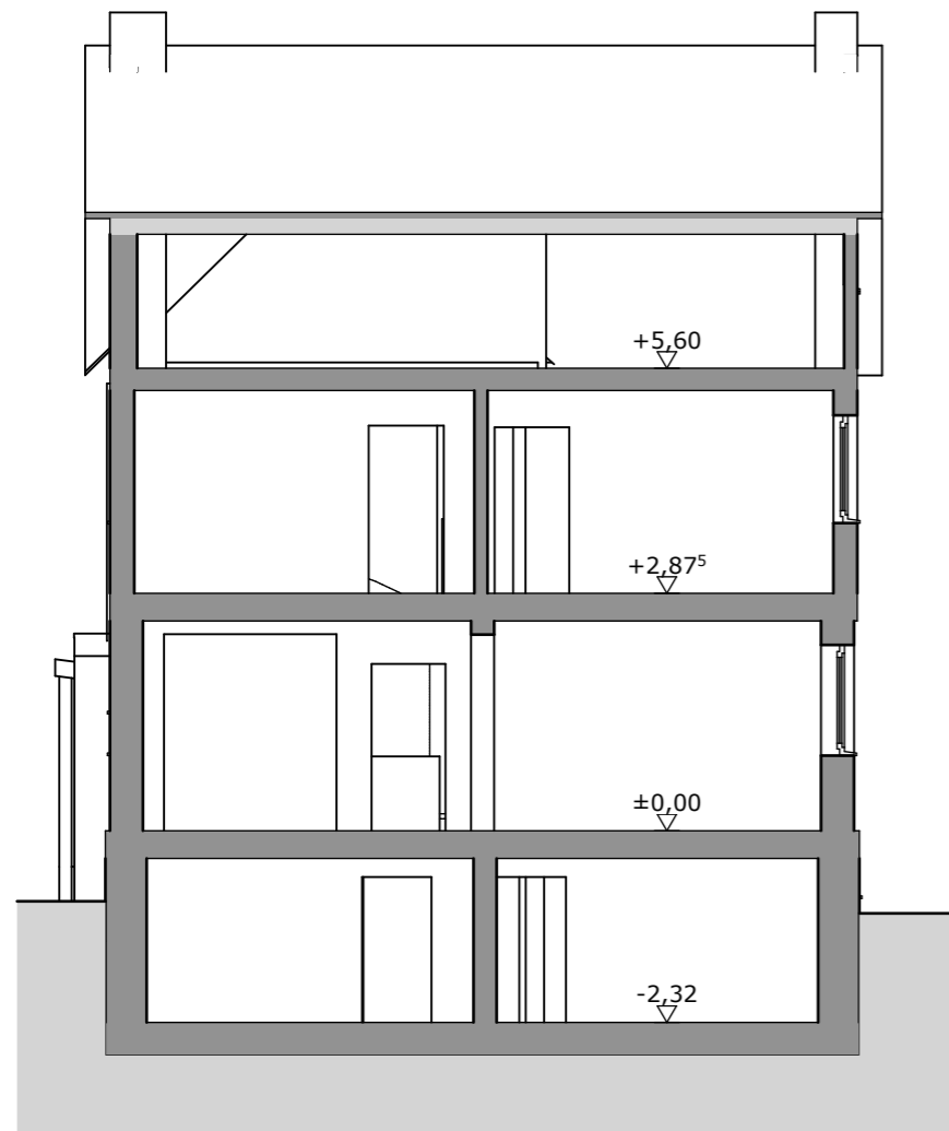
Schnitt B-B
